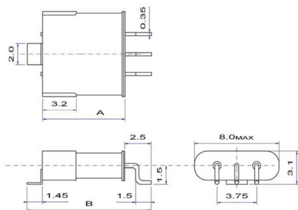
2 Poles & 4 Poles
